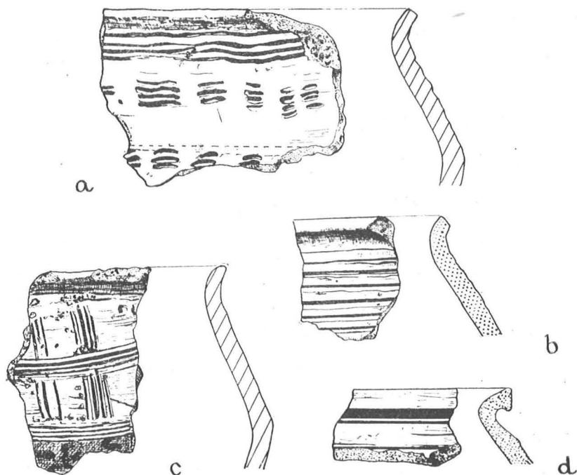
Ryc. 4. Topolno, pow. Świecie. Ceramika z warstwy I: (Skala 1:2) Fig. 4. Topolno, district of Swiecie. Pottery from layer I. (Scale 1:2).
