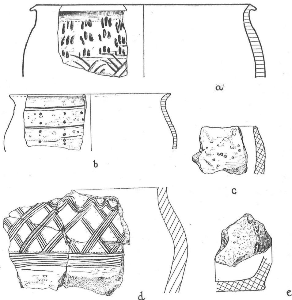
Ryc. 8. Topolno, pow. Świecie. Ceramika z warstwy IIa. (Skala 1:2) Fig. 8. Topolno, district of Świecie. Pottery from layer IIa. (Scale 1:2).
