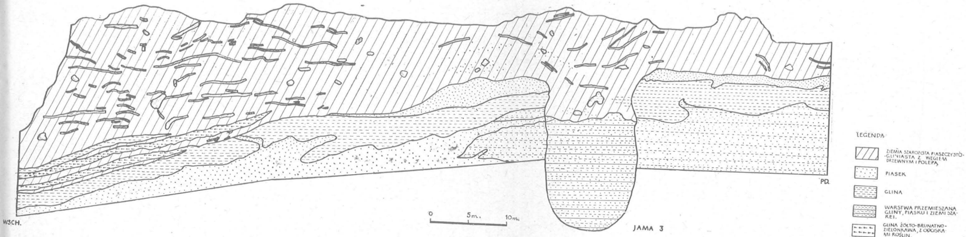
Tabl. IV. Topolno, pow. Świecie. Przekrój wału Table. IV. Topolno, district of Świecie. Section through the rampart.
