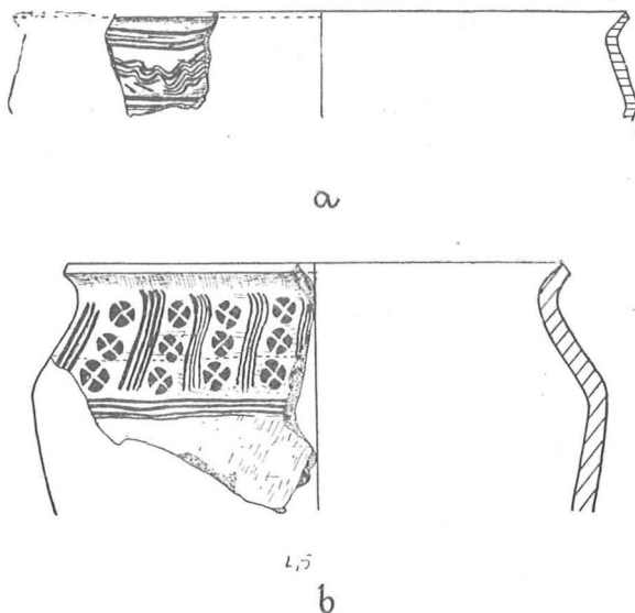
Ryc. 10. Topolno, pow. Świecie. Ceramika z warstwy IIa. (Skala 1:4) Fig. 10. Topolno, district of Świecie. Pottery from layer IIa (Scale 1:4).
