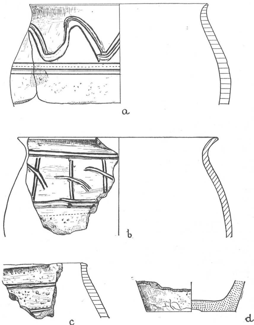
Ryc. 28. Topolno pow. Świecie. Ceramika z wału — z warstw IIb i III (Skala 1:2)
