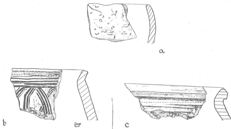
Ryc. 19. Topolno, pow. Świecie. Ceramika z jamy 1. (Skala 1:2) Fig. 19. Topolno, district of Świecie. Pottery from pit 1. (Scale 1:2).
