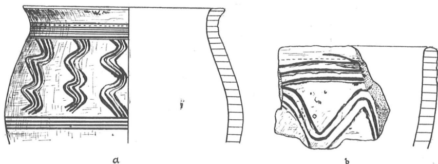
Ryc. 33. Topolno, pow. Świecie. Ceramika z jamy 5. (Skala 1:2)
