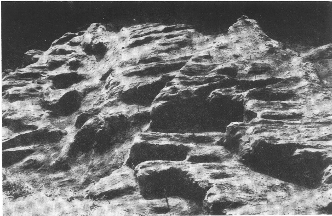
Ryc. 23. Topolno, pow. Świecie. Fragment 2 „warstewki” konstrukcji wału w stosie 3. (Fot. A. Kleina)
