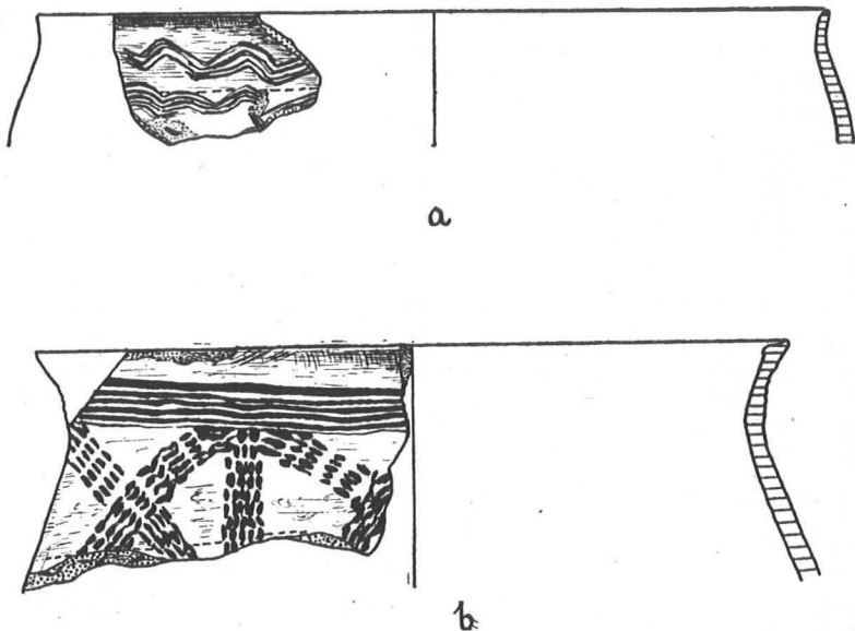
Ryc. 27. Topolno, pow. Świecie. Ceramika z wału — z warstw IIb i III. (Skala 1:4) Fig. 27. Topolno, district of Świecie. Pottery from rampart — from layers IIb and III (Scale 1:4)
