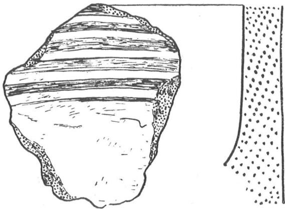
Ryc. 32. Topolno, pow. Świecie. Ceramika z warstwy IV. (Skala 1:1) Fig. 32. Topolno, district of Świecie. Pottery from layer IV (Scale 1:1)
