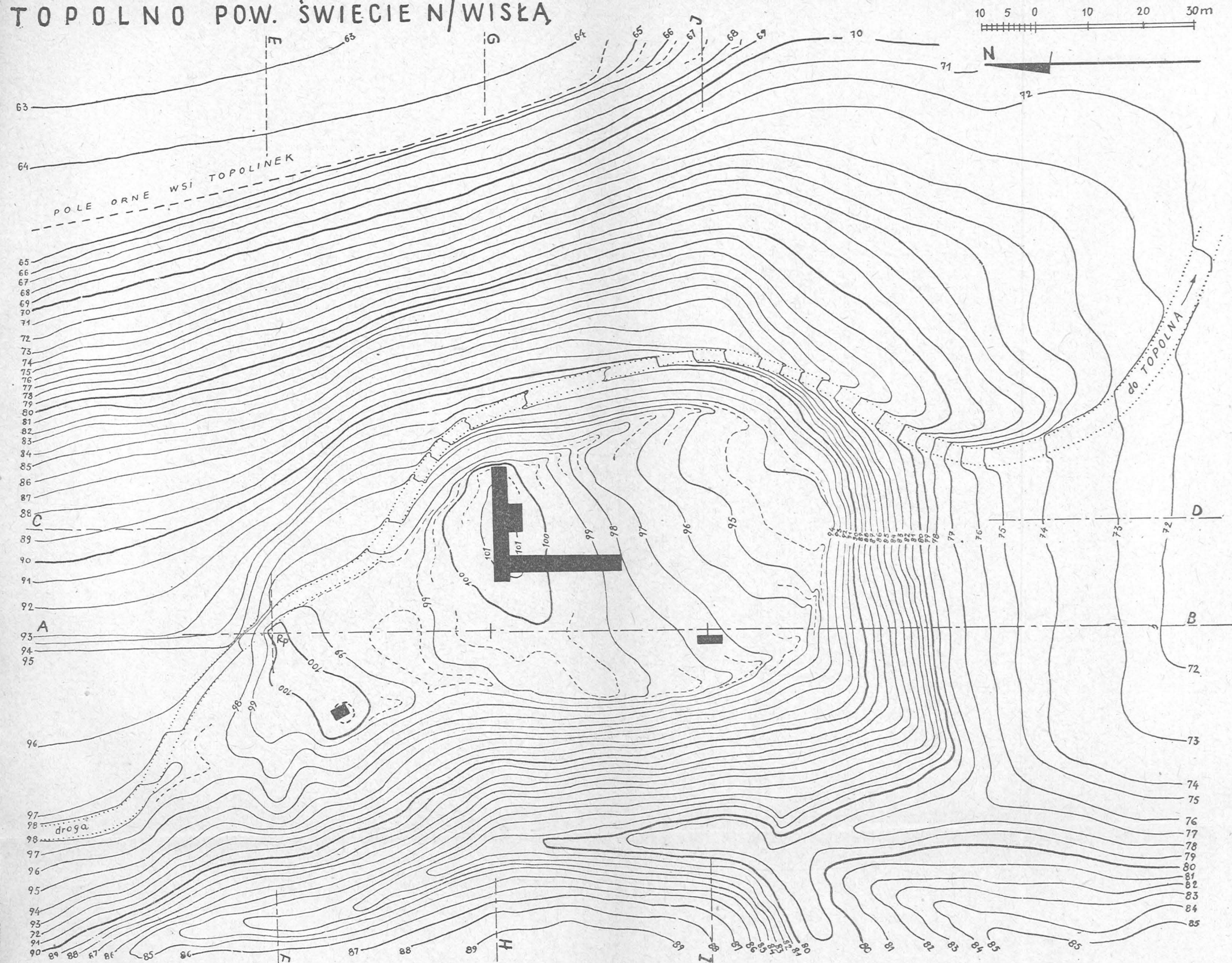
Tabl. I. Topolno, pow. Świecie. Plan warstwiczny grodziska z zaznaczeniem wykopów Table. I. Topolno, district of Świecie. Contour map of strong-hold with archaeological trenches marked.
