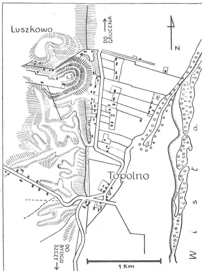
Ryc. 1. Topolno, pow. Świecie. Plan sytuacyjny grodziska Fig. 1. Topolno, district of Świecie. Site plan of the stronghold.
