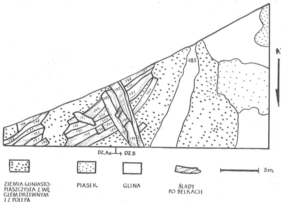
Ryc. 24. Topolno, pow. Świecie. 25 „warstewka” konstrukcji wału w stosie 2. Fig. 24. Topolno, district of Świecie. 25th thin layer with rampart remains in pile 2.
