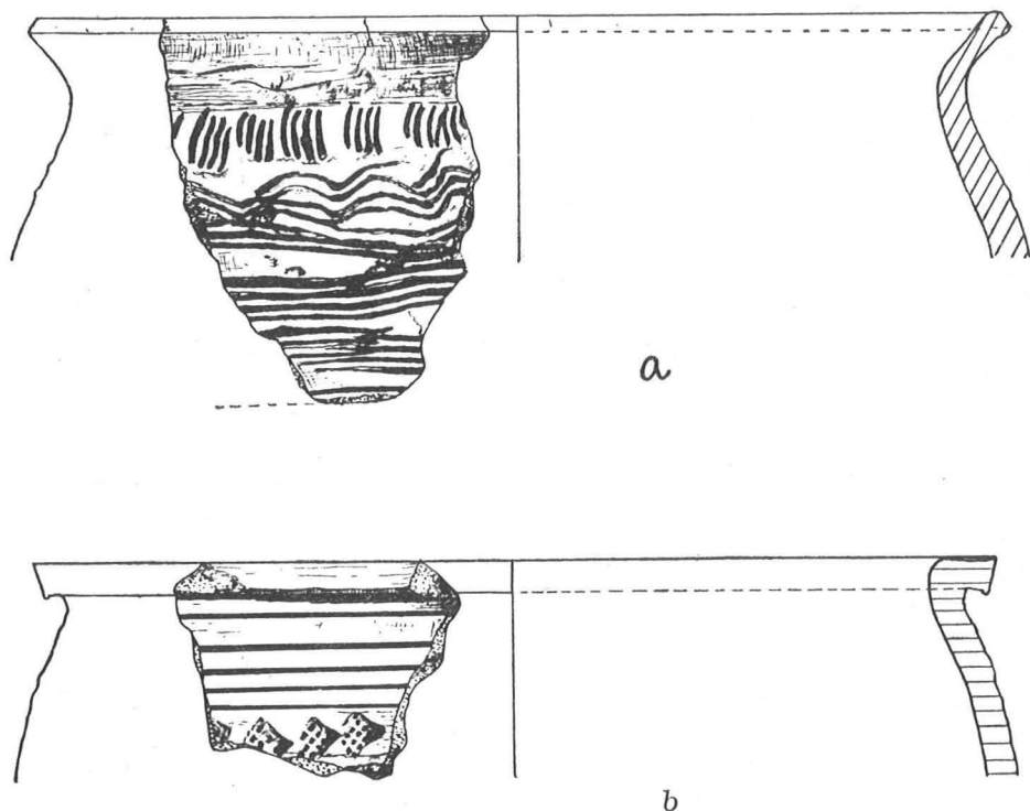
Ryc. 12. Topolno, pow. Świecie. Ceramika z warstwy IIa. (Skala 1:2) Fig. 12. Topolno, district of Świecie. Pottery from layer IIa (Scale 1:2).
