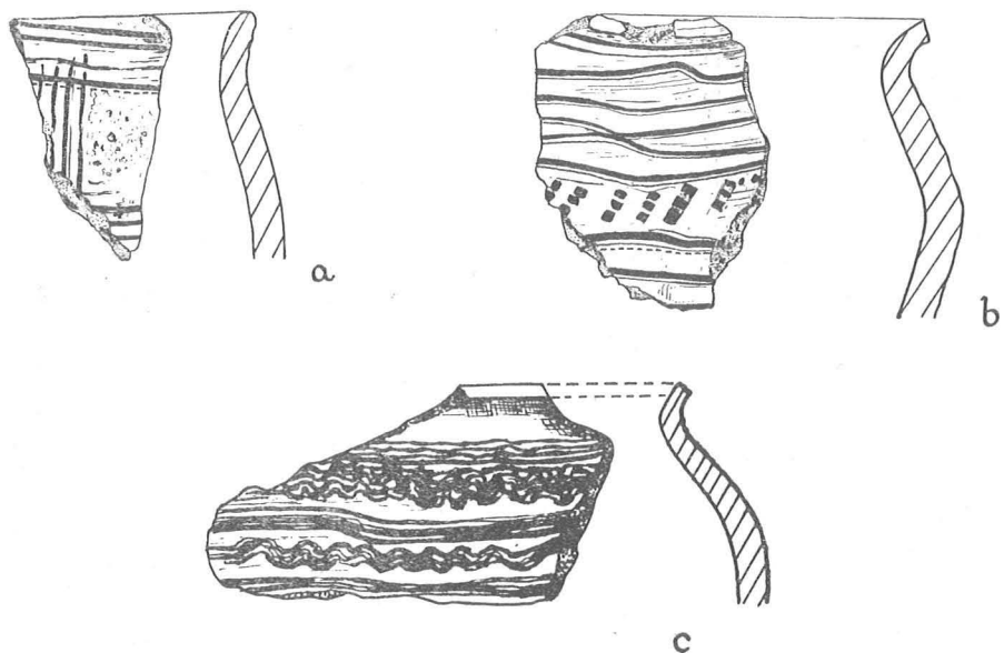
Ryc. 17. Topolno, pow. Świecie. Ceramika z paleniska 1. (Skala 1:2) Fig. 17. Topolno, district of Świecie. Pottery from hearth 1 (Scale 1:2).
