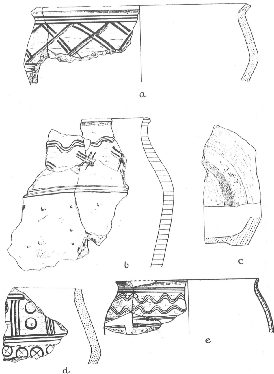
Ryc. 29. Topolno, pow. Świecie. Ceramika z wału — z warstw IIb i III (Skala: a — d — 1:2, e — 1:4)
