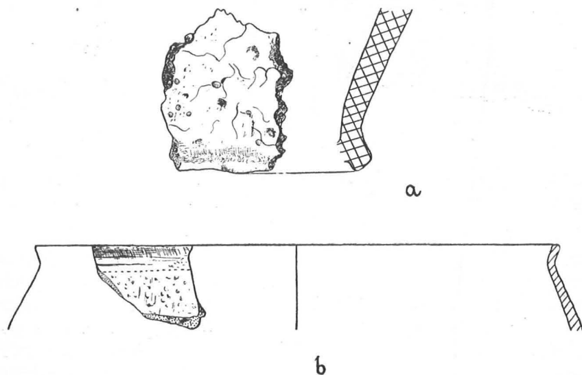
Ryc. 26. Topolno, pow. Świecie. Ceramika z wału — z warstw IIb i III (Skala: a — 1:2, b — 1:4)
