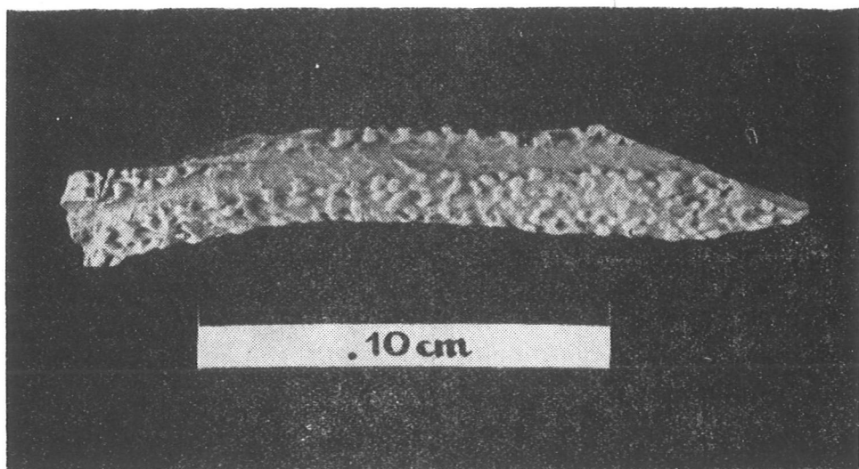
Ryc. 21. Topolno, pow. Świecie. Przedmiot rogowy z jamy 4. (Fot. A. Kleina)
