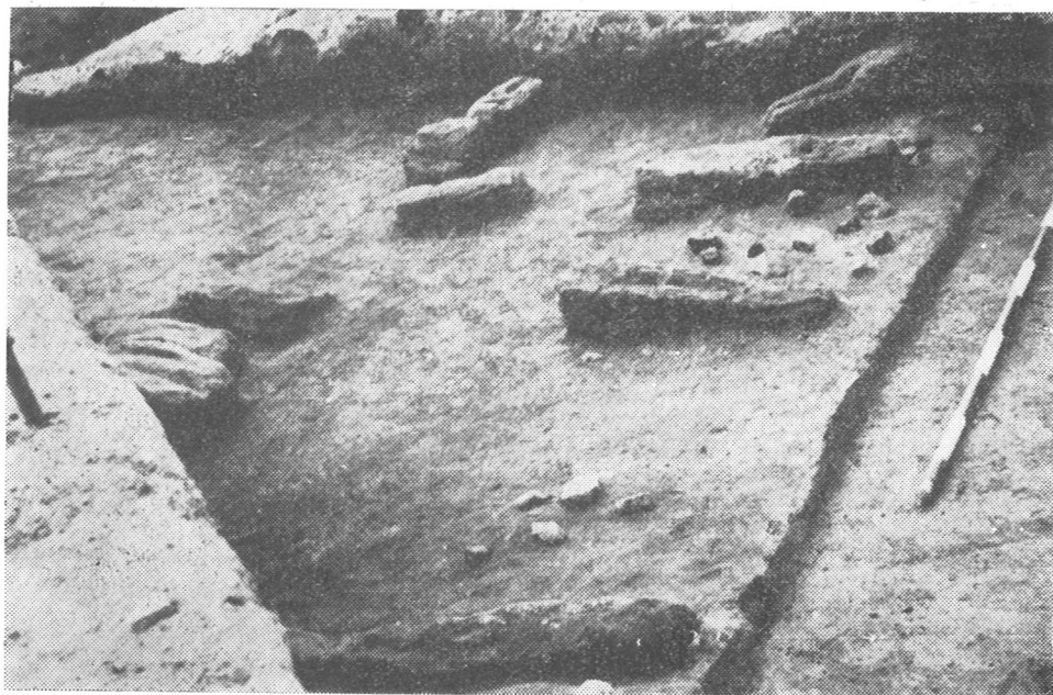
Ryc. 22. Topolno, pow. Świecie. Najlepiej zachowana „warstewka” konstrukcji wału w stosie 4. (Fot. H. Późniak)
