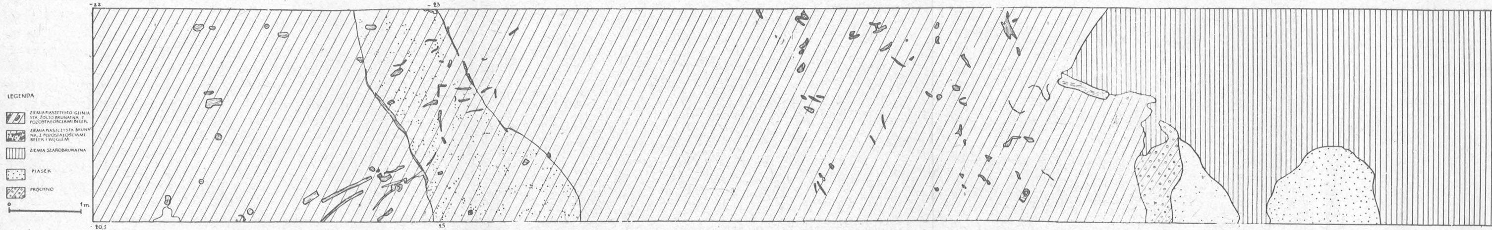
Tabl. II. Topolno, pow. Świecie. Rzut poziomy warstw: IIa, IIb i IIc w wykopie I Table II. Topolno, district of Świecie. Ground plan of layers: IIa, IIb and IIc in trench I.
