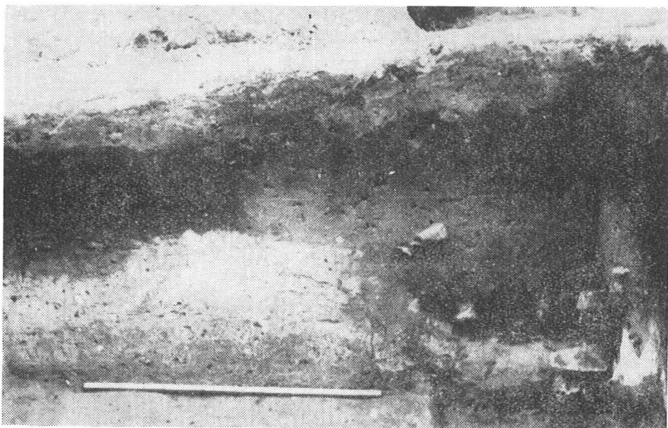
Ryc. 16. Topolno, pow. Świecie. Palenisko 1 i jama 2 w profilu północnym działki A wykopu III. (Fot. A. Późniak)
