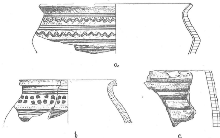
Ryc. 20. Topolno, pow. Świecie. Ceramika z jamy 4. (Skala 1:3) Fig. 20. Topolno, district of Świecie. Pottery from pit 4. (Scale 1:3).
