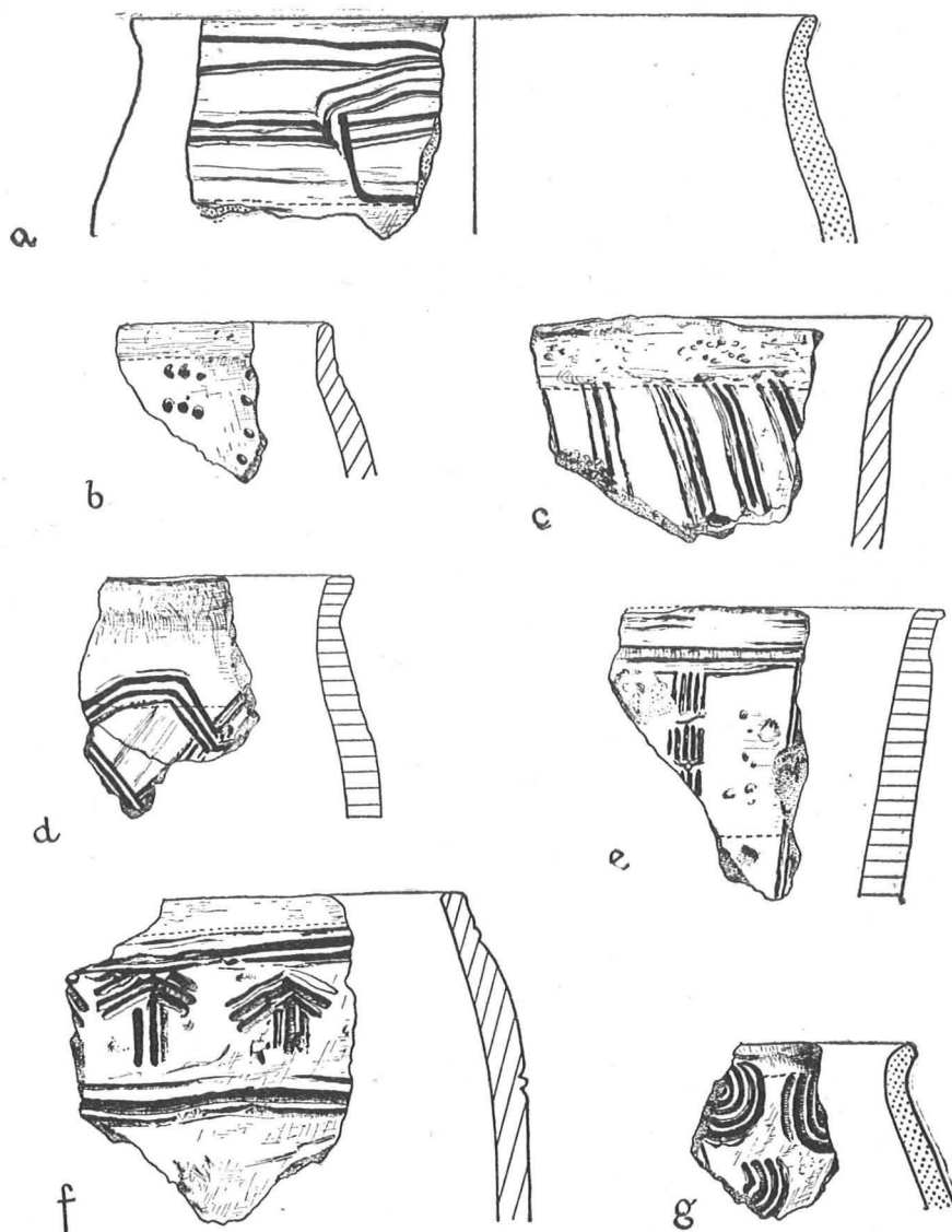
Ryc. 7. Topolno, pow. Świecie. Ceramika z warstwy IIa. (Skala 1:2) Fig. 7. Topolno, district of Świecie. Pottery from layer IIa (Scale 1:2).
