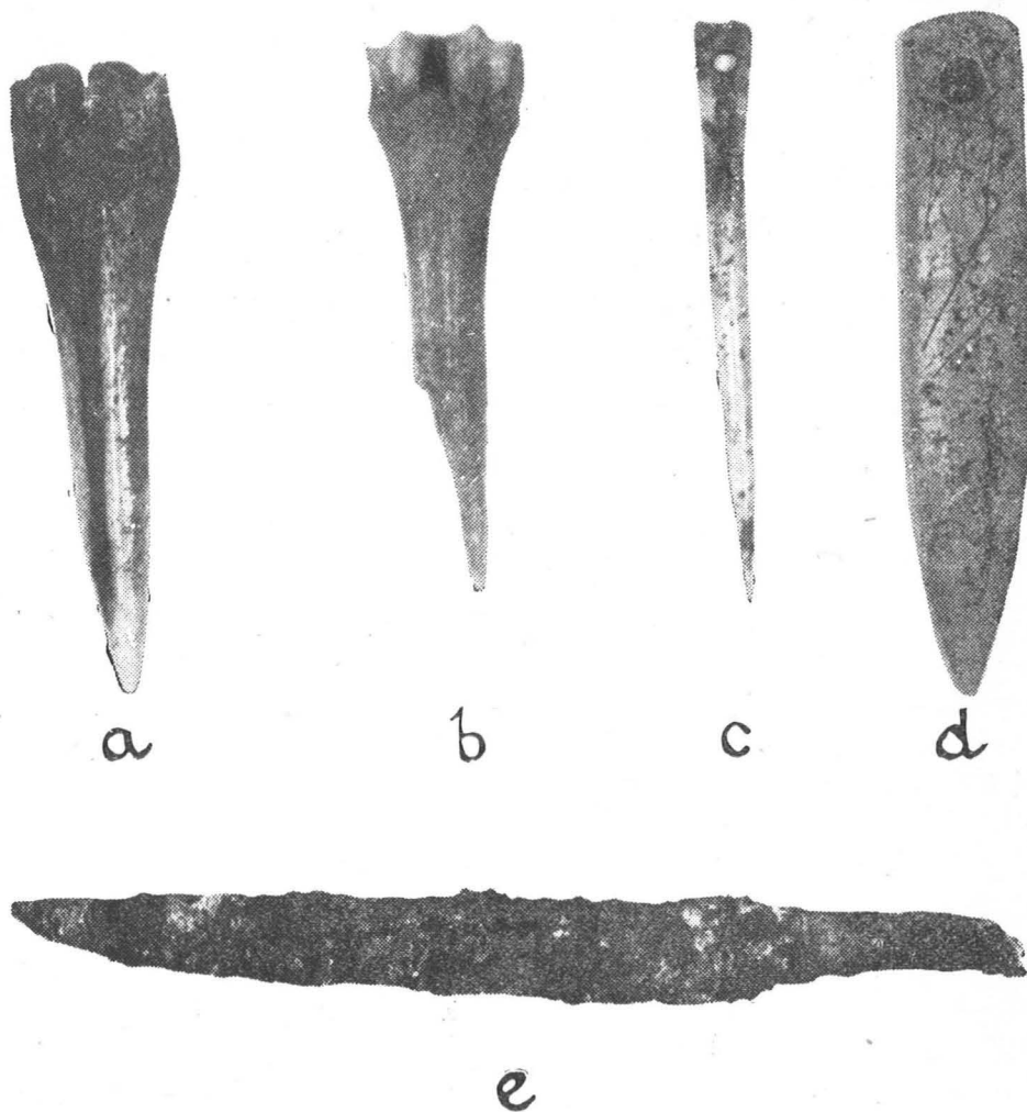
Ryc. 15. Topolno, pow. Świecie. Zabytki z warstwy IIa, a, b — szydła kościane, c, d — igły kościane, e — nożyk żelazny. (Skala 1:1). Fot. A. Kleina
