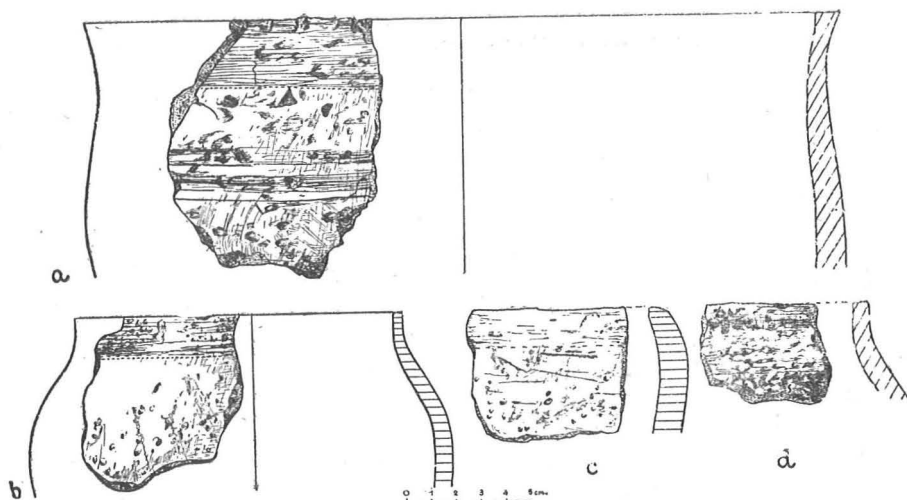
Ryc. 6. Topolno, pow. Świecie. Ceramika z warstwy IIa. (Skala 1:3)
