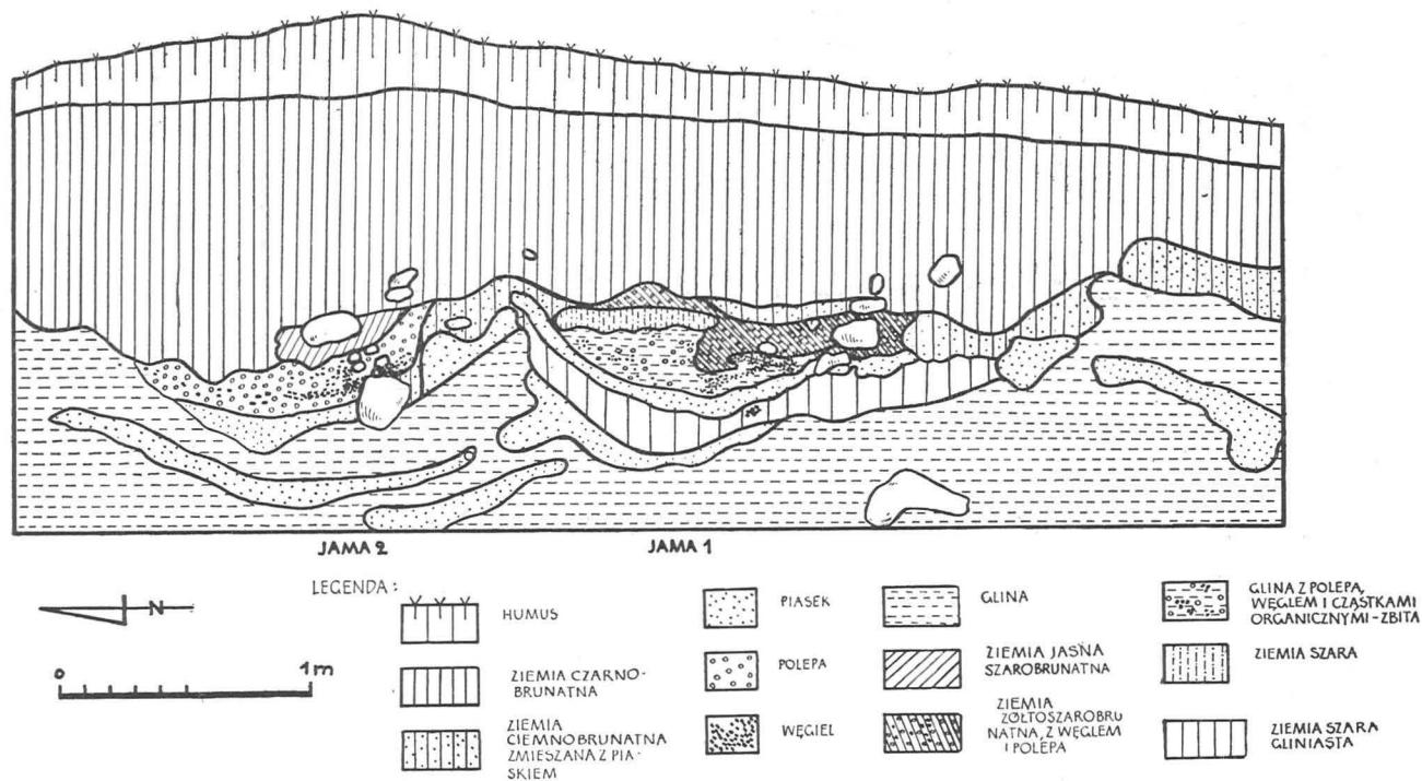
Ryc. 18. Topolno, pow. Świecie. Jama 1 i 2 w profilu wschodnim działki A wykopu III Fig. 18. Topolno, district of Świecie. Pit 1 and 2 in eastern cutting of section A in trench III.
