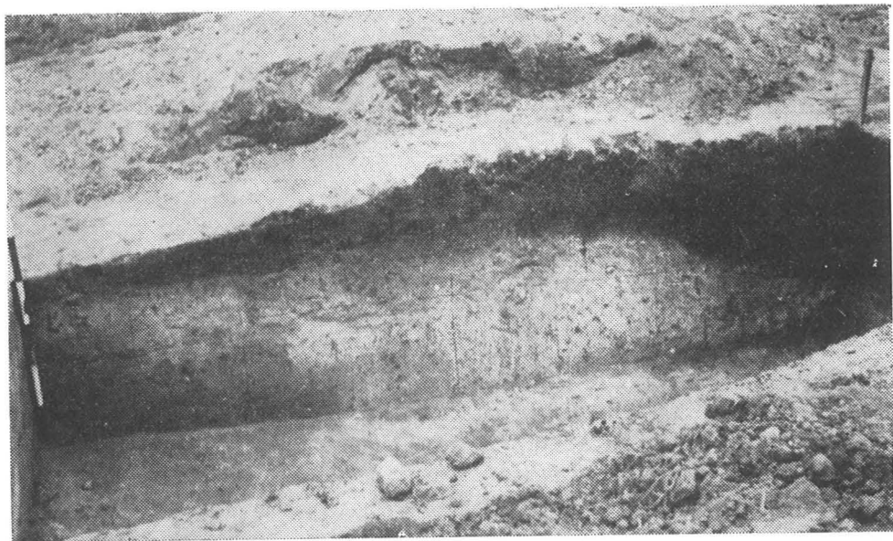
Ryc. 5. Topolno, pow. Świecie. Warstwa IIa w zachodnim profilu działki A wykopu III. (Fot. H. Późniak)
