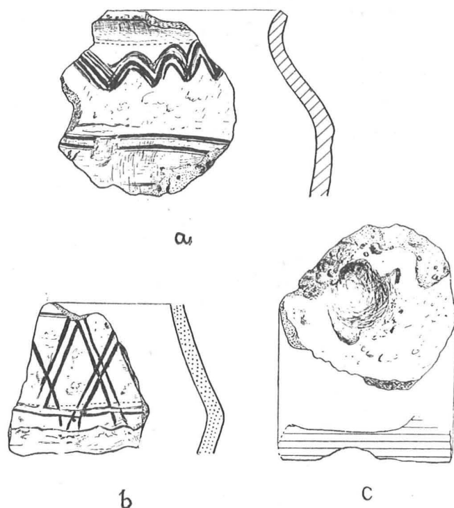
Ryc. 11. Topolno, pow. Świecie. Ceramika z warstwy IIa. (Skala 1:2) Fig. 11. Topolno, district of Świecie. Pottery from layer IIa (Scale 1:2).
