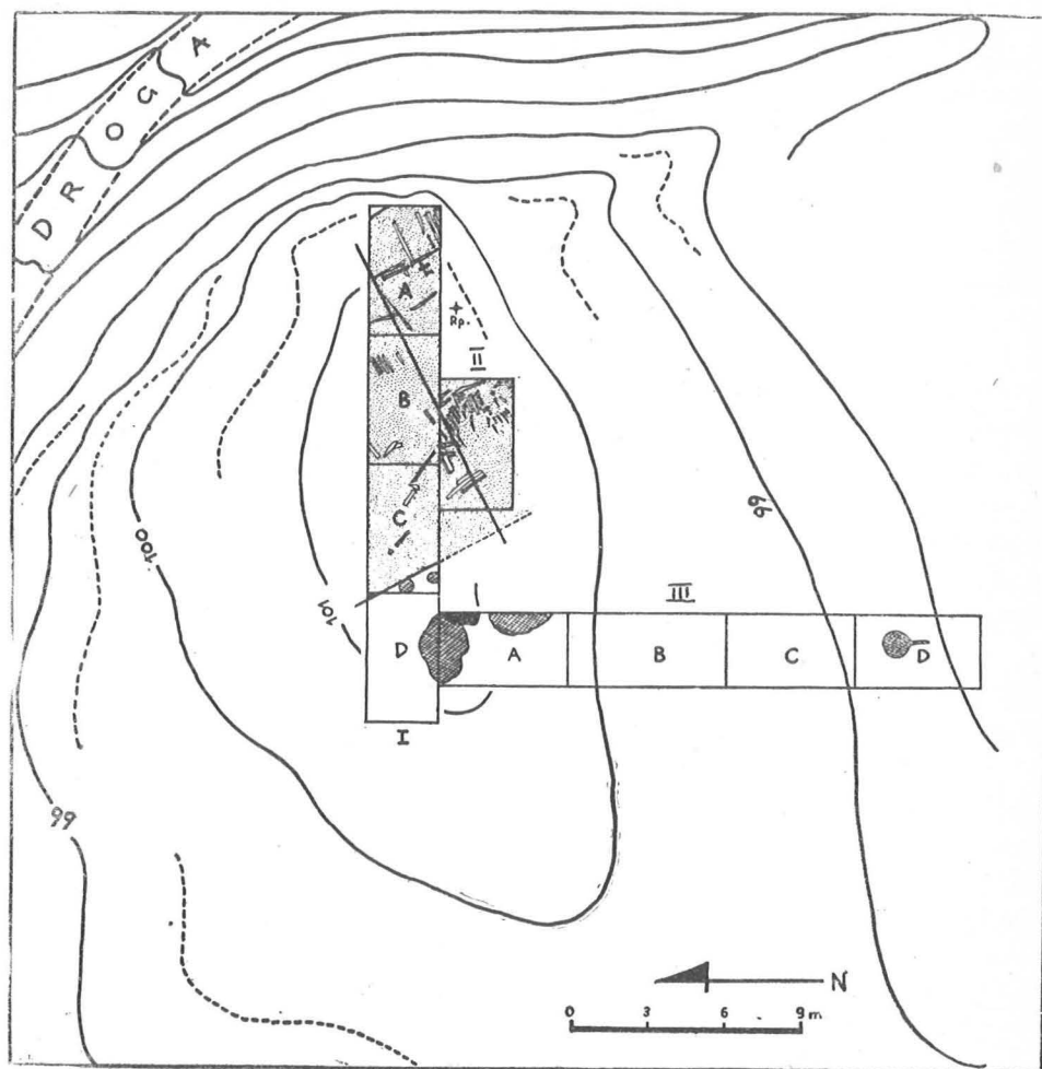
Ryc. 3. Topolno, pow. Świecie. Plan sytuacyjny wykopów na grodzisku Fig. 3. Topolno, district of Świecie. Site plan of trenches in the stronghold.
