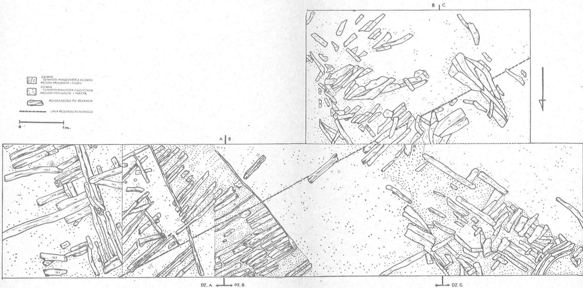
Tabl. III. Topolno, pow. Świecie. Rzut poziomy 2 „warstewki” konstrukcji wału w wykopie I i II Table III. Topolno, district of Świecie. Ground plan of second thin layear with rampart remains in trench I and II.
