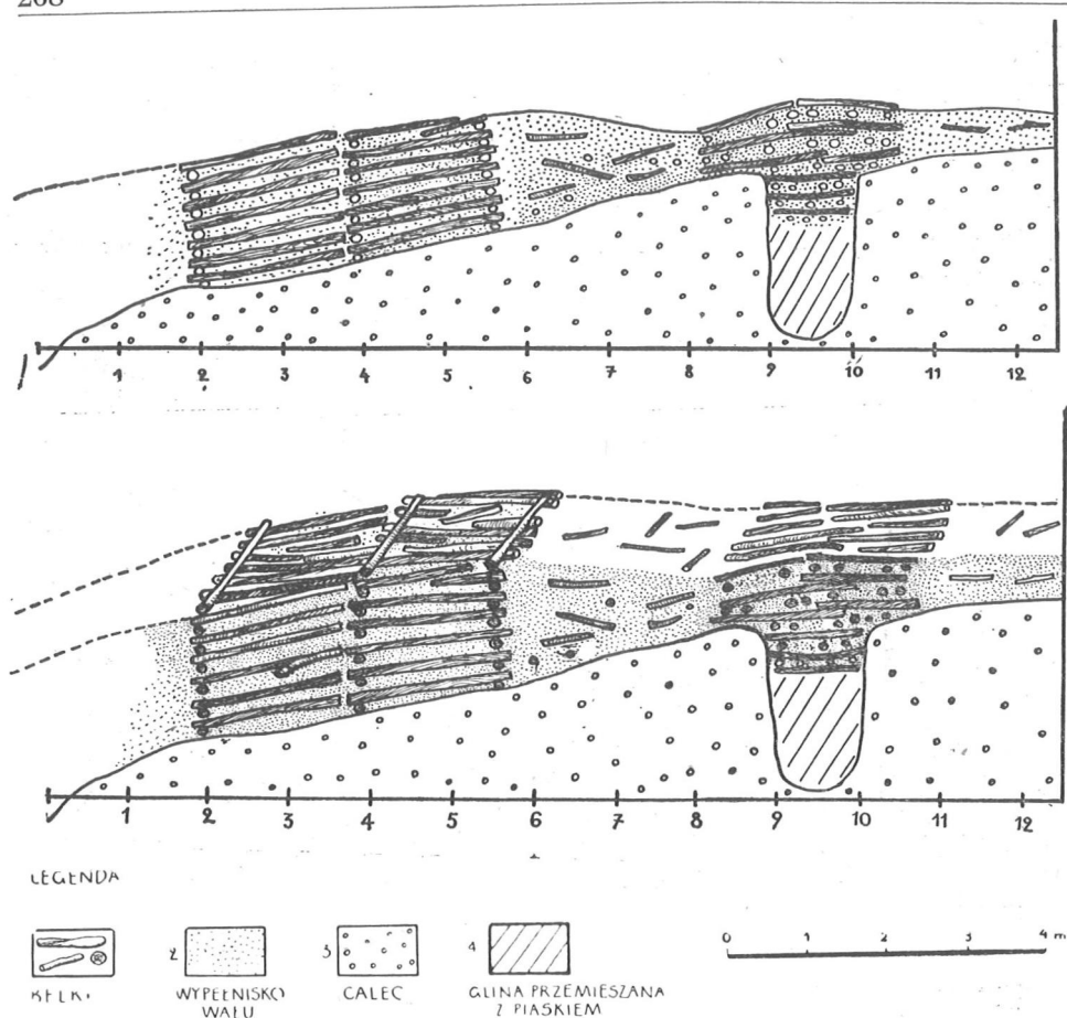
Ryc. 25. Topolno, pow. Świecie. Próba rekonstrukcji wału.
