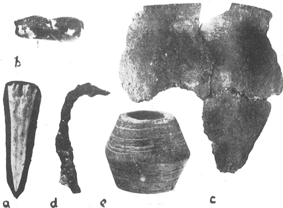
Ryc. 30. Topolno, pow. Świecie. Zabytki z wału — z warstw IIb: a — szydło kościane, b — paciorek szklany, c — fragment naczynia, d — haczyk żelazny, e — przesłik gliniany. (Skala: a, c — 1:2; b, d, e — 1:1). (Fot. A. Kleina)
