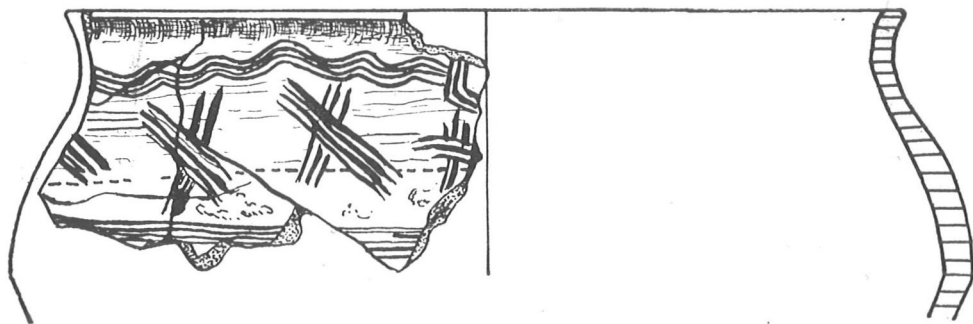
Ryc. 31. Topolno, pow. Świecie. Ceramika z warstwy IIc. Fig. 31. Topolno, district of Świecie. Pottery from layer IIc.
