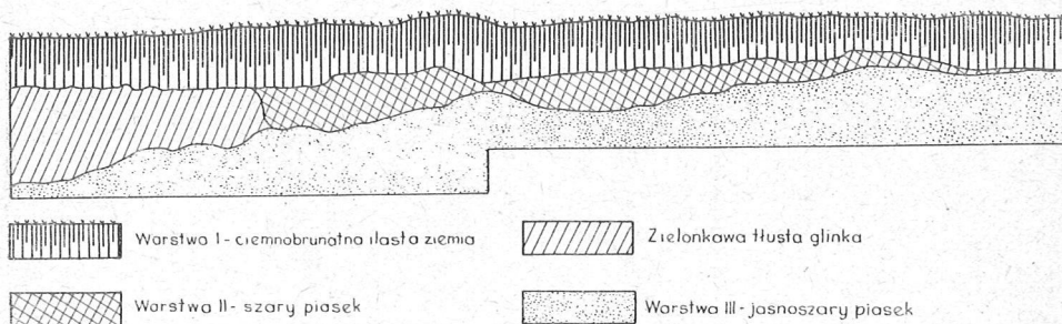
Ryc. 3. Lichnowy, pow. Malbork, profil północny wykopu z widocznymi trzema warstwami, skala 1 : 100
