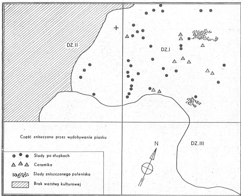
Ryc. 4. Lichnowy, pow. Malbork, rzut poziomy wykopu z zaznaczonymi śladami po słupkach i częścią wykopu (dz. II), gdzie nie wystąpiła warstwa kulturowa, skala 1 : 80.
