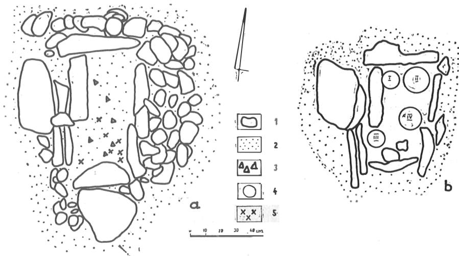
Ryc. 13. Gościcino, pow. Wejherowo, st. 3. Rzuty poziome grobu nr 12: a — wierzch grobu z rysującą się skrzynią grobową, b — wnętrze skrzyni grobowej wraz z popielnicami
