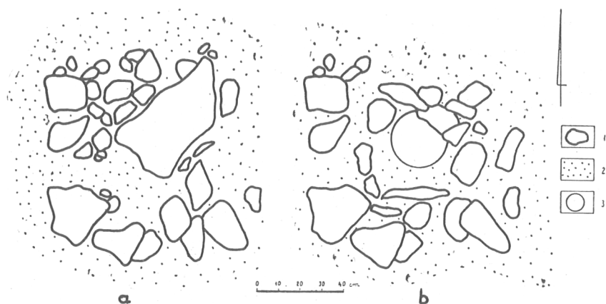
Ryc. 28. Gościcino, pow. Wejherowo, st. 3. Rzuty poziome grobu nr 27: a — dno grobu, b — popielnica otoczona obwarowaniem
