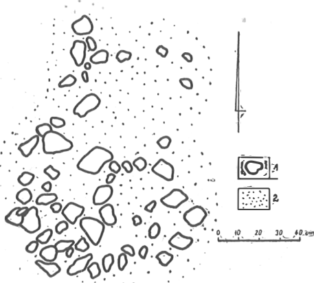
Ryc. 29. Gościcino, pow. Wejherowo, st. 3. Rzut poziomy grobu nr 28
