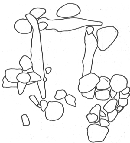
Ryc. 14. Gościcino, pow. Wejherowo, st. 3. Rzut poziomy grobu nr 13, poniżej rzut i przekrój jamy zawierającej spaleniznę i węgielki drzewne
