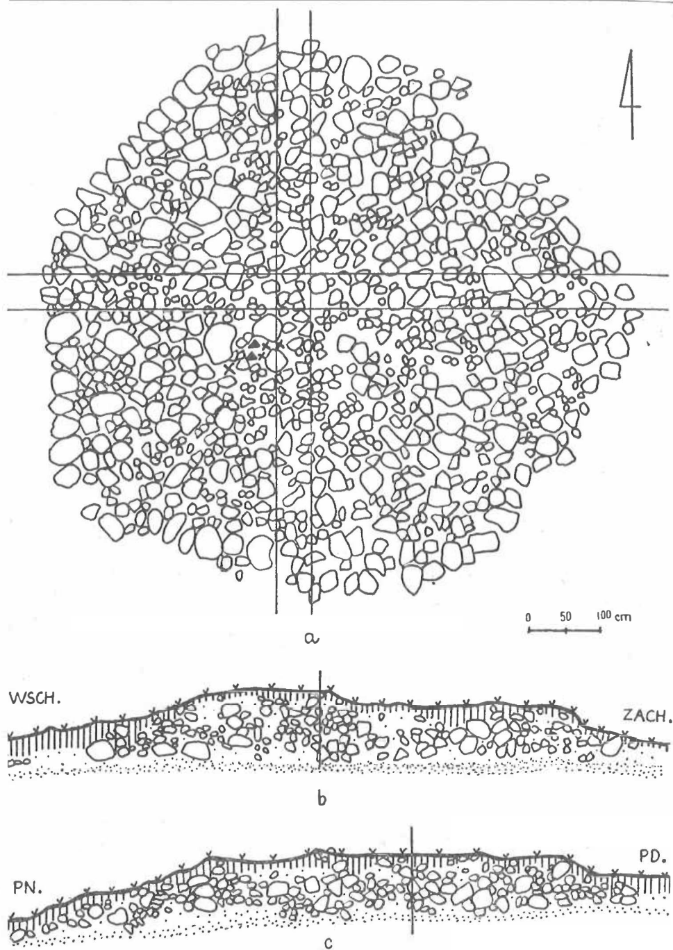
Ryc. 5. Siemirowice, gm. Cewice, st. 1. Kurhan I: a — płaszcz kamienny, b, c — profile na osi wsch.-zach. i pñ.-płd.
