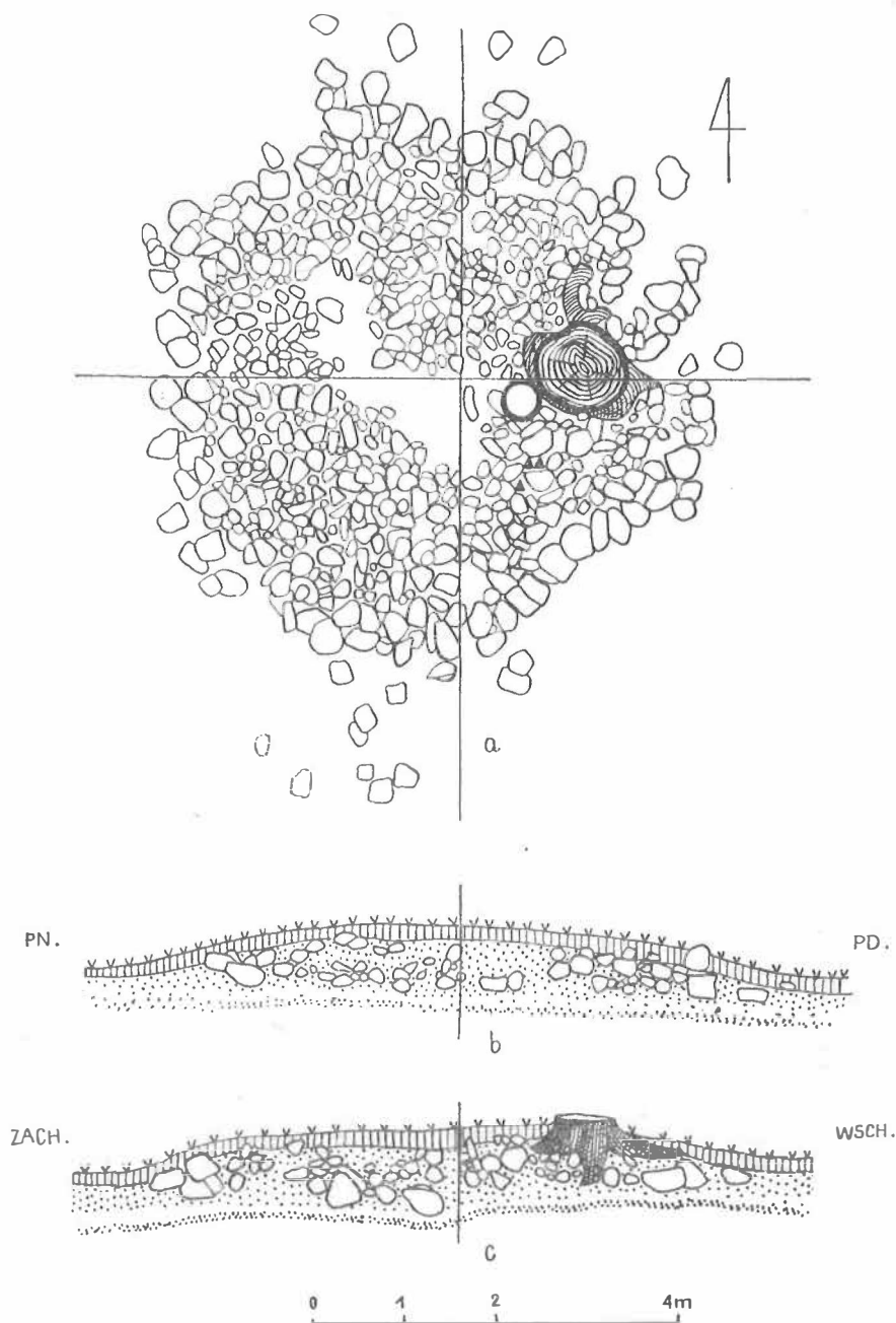
Ryc. 39. Siemirowice, gm. Cewice, st. 1. Kurhan XXIV: a — płaszcz kamienny, b, c — profile na osi wsch.-zach. i płn.-płd.
