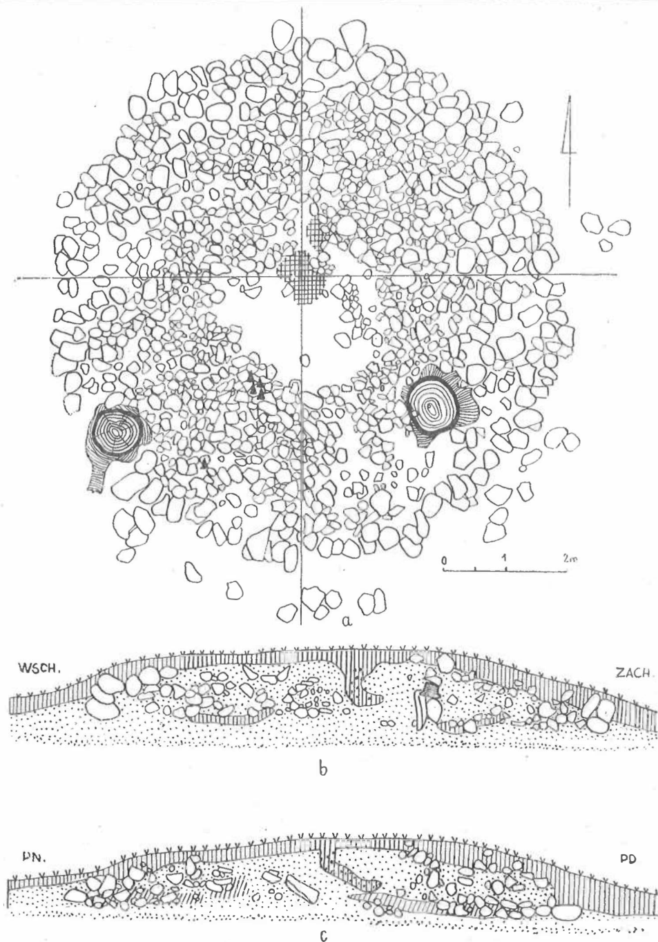
Ryc. 25. Siemirowice, gm. Cewice, st. 1. Kurhan XX: a — płaszcz kamienny, b, c — profile na osi wsch.-zach. i półn.-półd.
