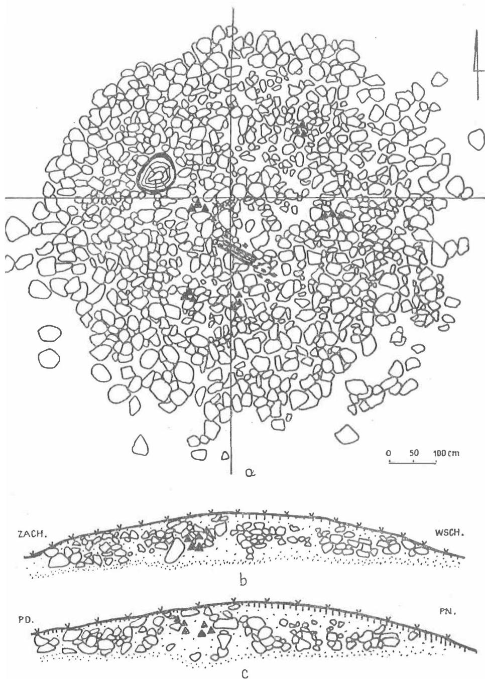
Ryc. 42. Siemirowice, gm. Cewice, st. 1. Kurhan XXVI, a — płaszcz kamienny, b, c — profile na osi wsch.-zach. i półn.-półd.
