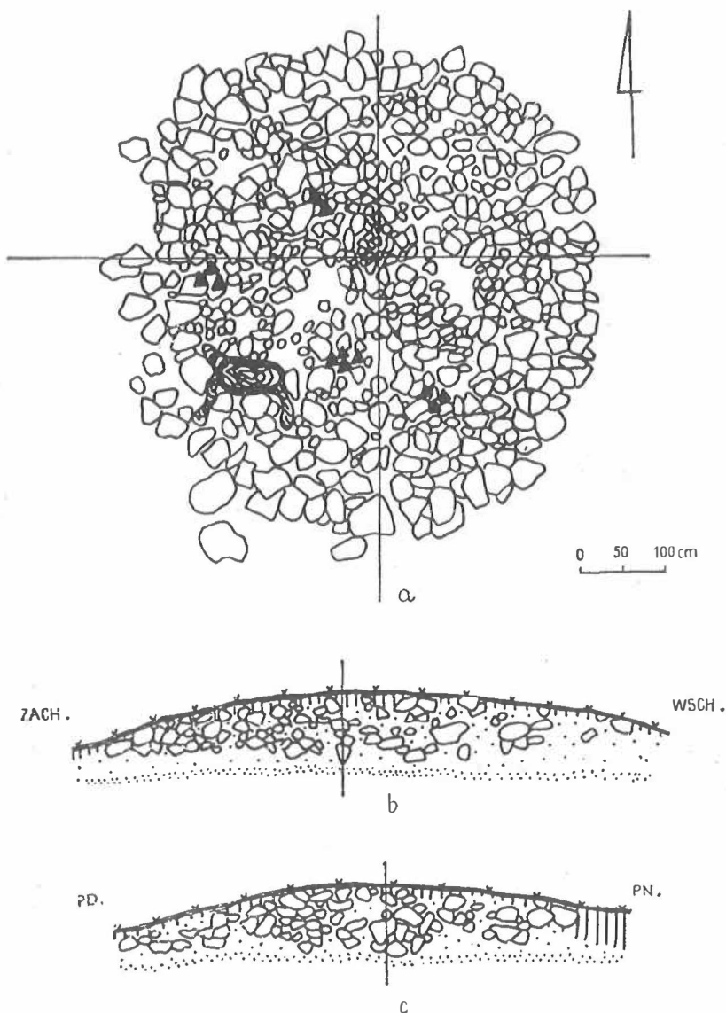
Ryc. 30. Siemirowice, gm. Cewice, st. 1. Kurhan XXI: a — płaszcz kamienny b, c — profile na osi wsch.-zach. i płn.-płd.
