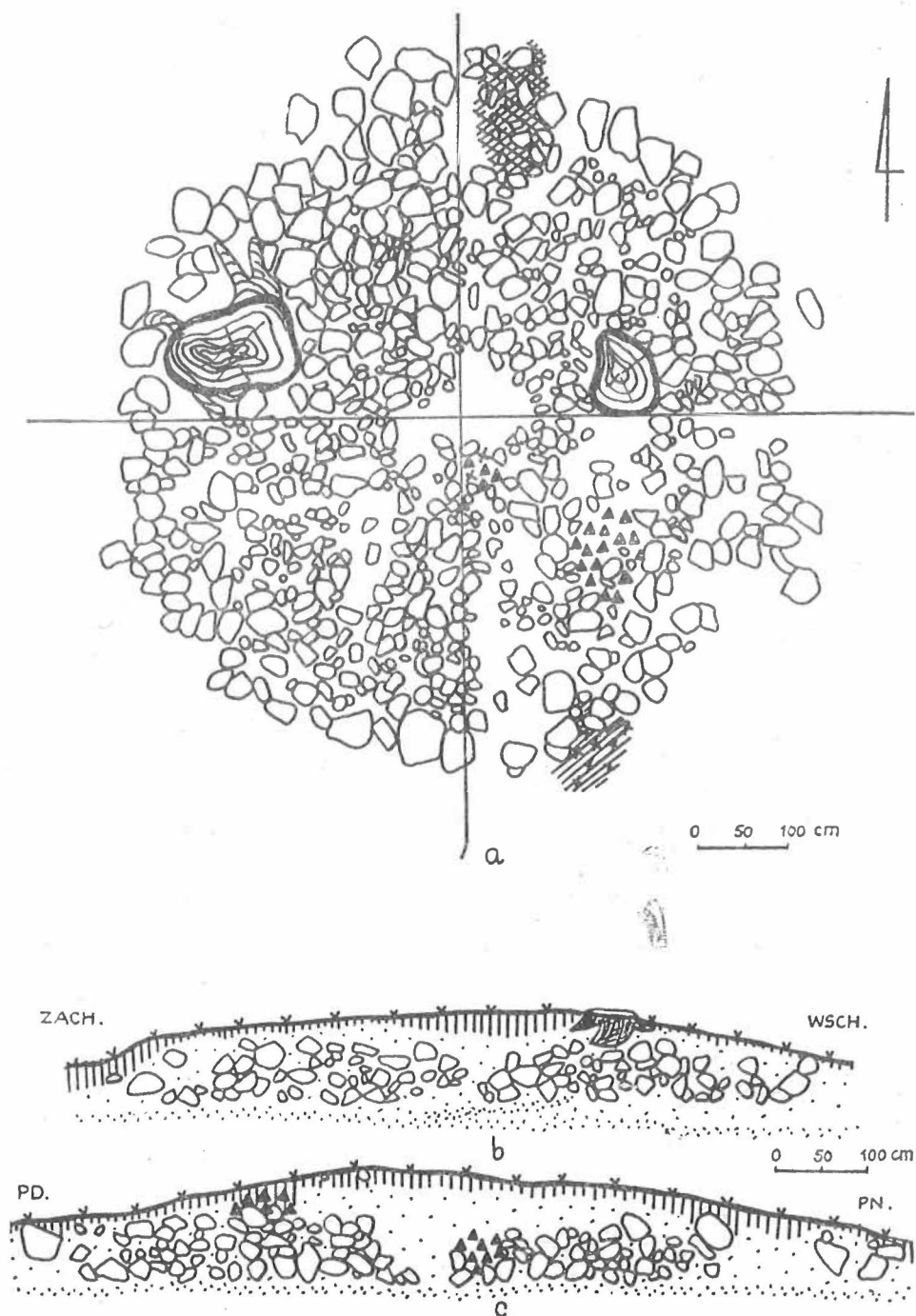
Ryc. 51. Siemirowice, gm. Cewice, st. 1. Kurhan XLV: a — płaszcz kamienny, b, c — profile na osi wsch.-zach. i pñ.-płd.
