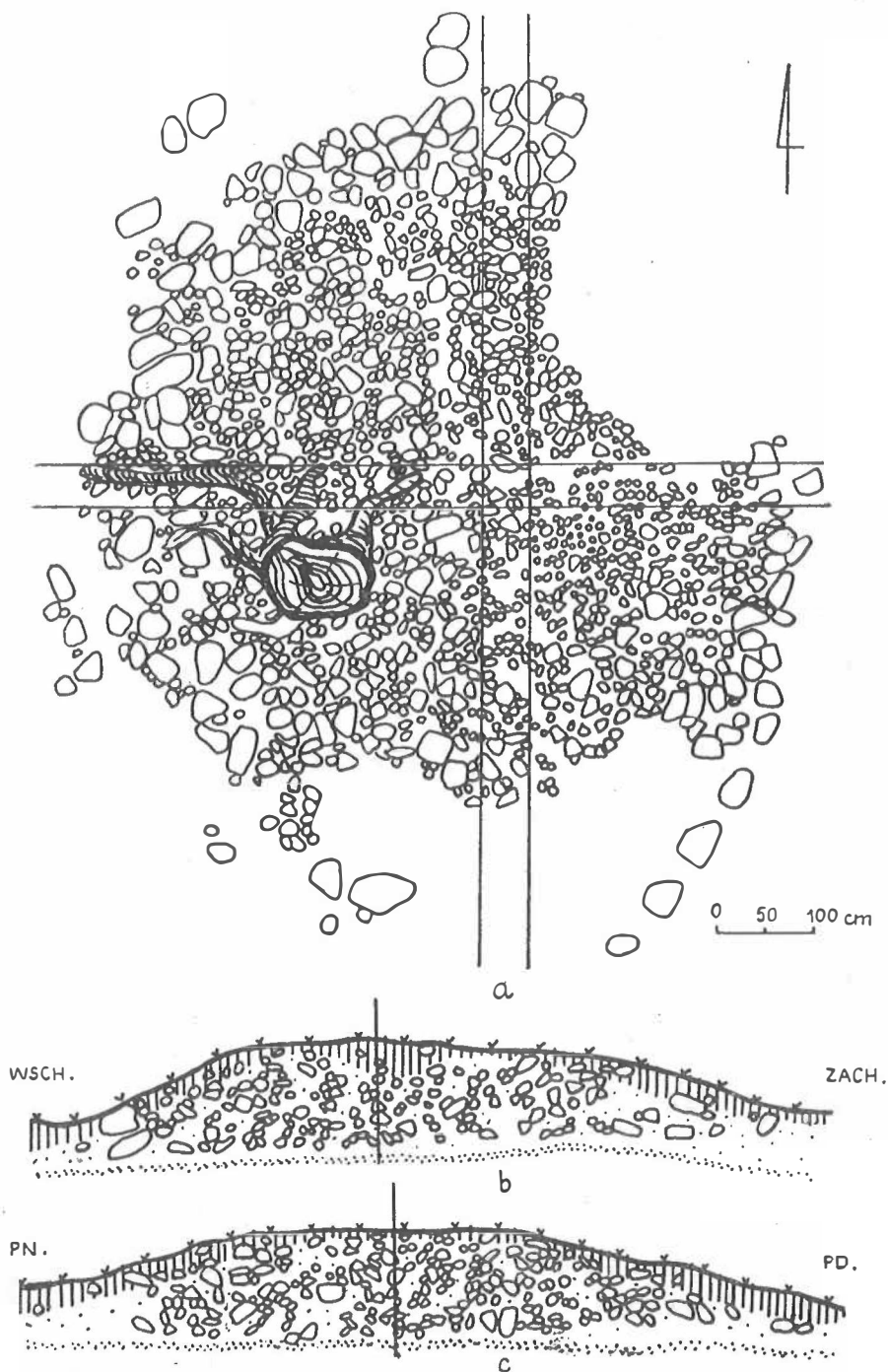
Ryc. 23. Siemirowice, gm. Cewice, st. 1. Kurhan XIII, a — płaszcz kamienny, b, c — profile na osi wsch.-zach. i póln.-płd.
