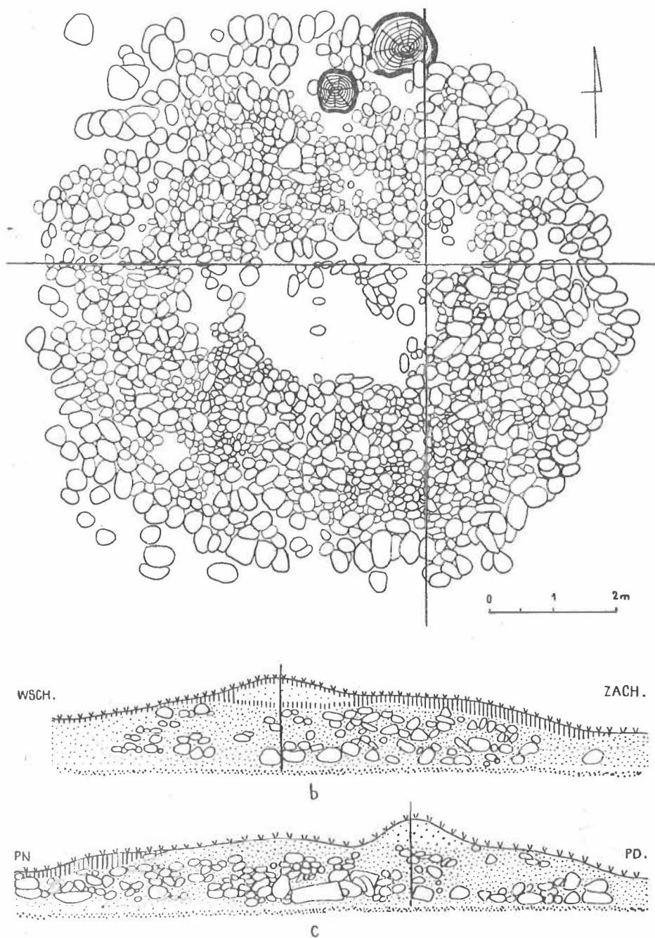
Ryc. 32. Siemirowice, gm. Cewice, st. 1. Kurhan XXII: a — płaszcz kamienny, b, c — profile na osi wsch.-zach. i półn.-półd.
