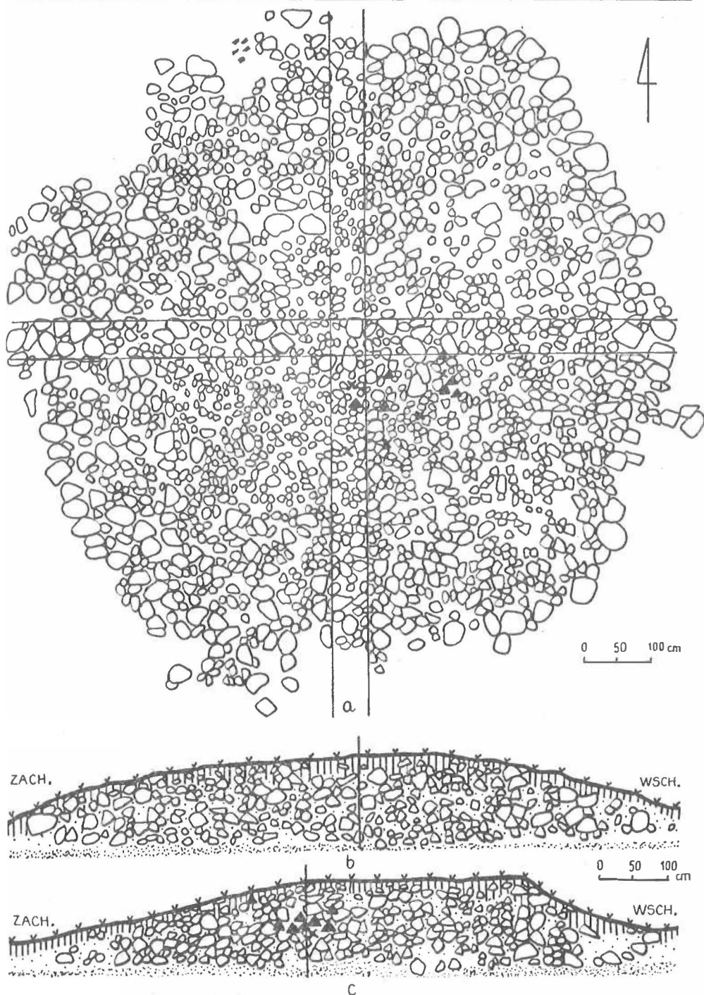
Ryc. 8. Siemirowice, gm. Cewice, st. 1. Kurhan II: a — płaszcz kamienny, b, c — profile kurhanu na osi wsch.-zach. i pñ.-płd.
